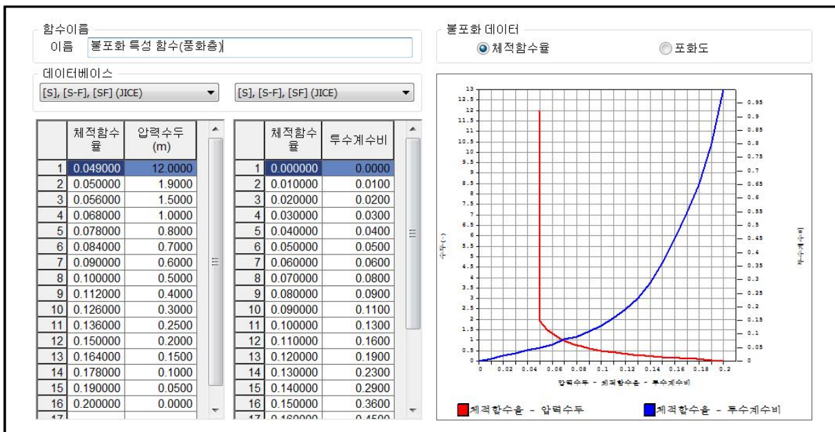
<그림 27-15> 압력수두-체적함수(포화도)-투수계수비 함수
